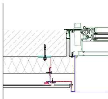
OPCIÓN CON ALUMINIO LACADO PAINTED ALUMINIUM OPTION
