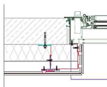
OPCIÓN CON REVEST.CERÁMICO CERAMIC OPTION
